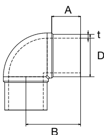
Угольник 90° PP-RCT, S 5 / SDR 11
