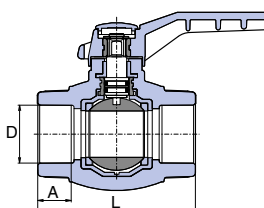
Шаровой кран
