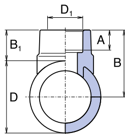
Вварное седло
